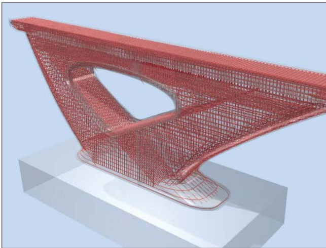
Mit einem 3D-Bewehrungsmodell erkennen Sie Konflikte bereits während der Planung. (Vorgespannter Autobahnbrückenpfeiler bei Haarlem, Iv-Infra, Nieuwegein, NL)
