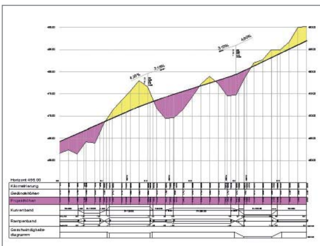
Lageplan, Höhenplan und Querprofile werden aus dem 3D-Modell abgeleitet. (Höhenplan Zufahrtsstraße Payerne, Département des Infrastructures, Lausanne, CH)
