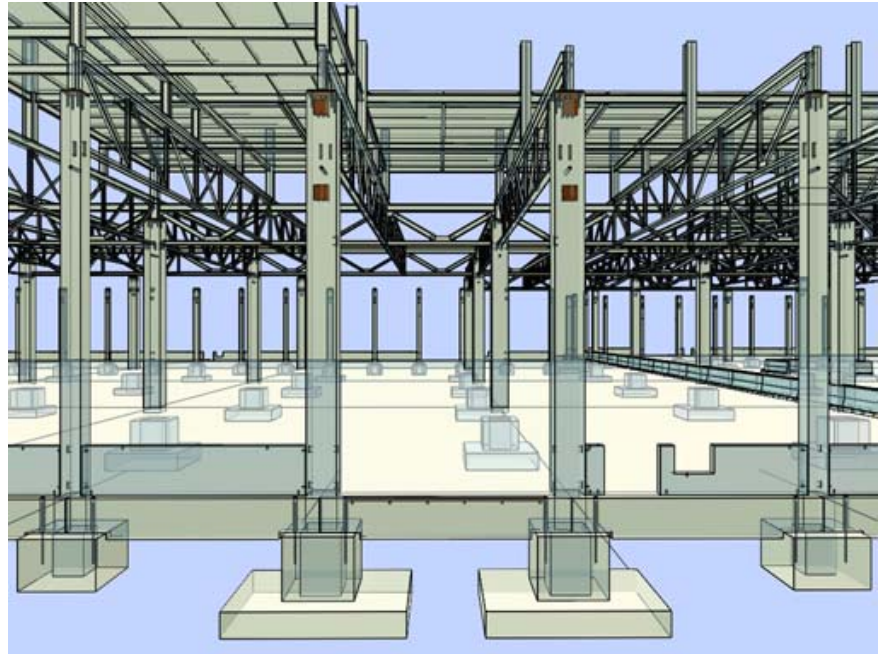
Supplier Park, Ingenieurbüro Aloys Kerber, Merzig
