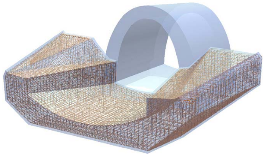
Einlaufbauwerk, Baukonstruktion Wolf, Berlin
